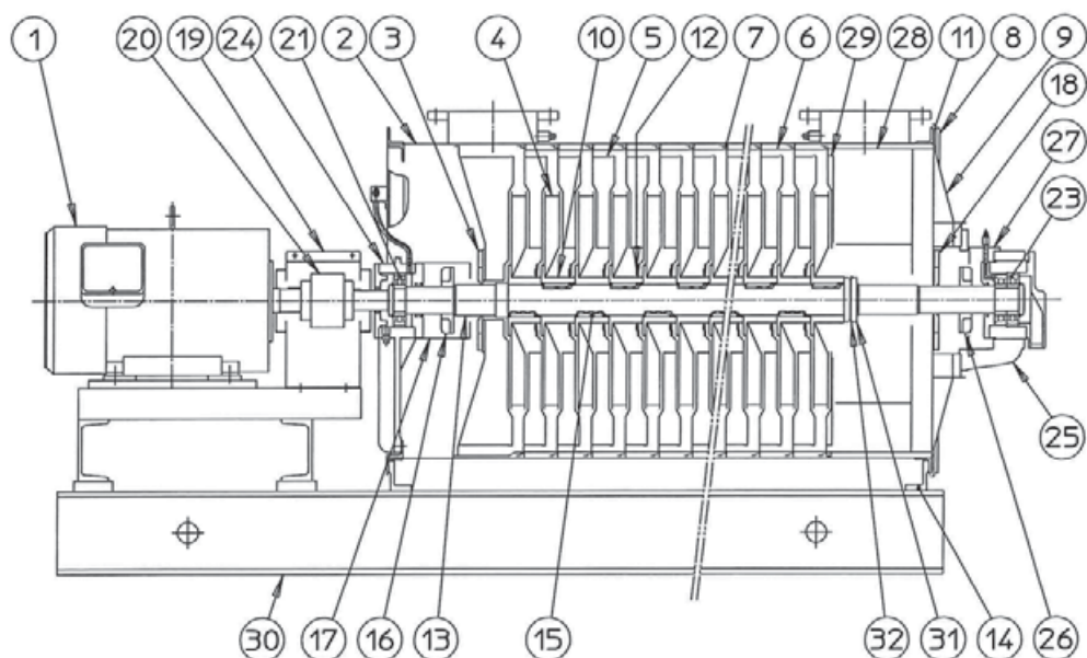
4BOBタイプ（直結形）構造断面図
