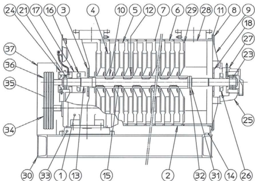
4BOBタイプ（ベルト駆動形）構造断面図
